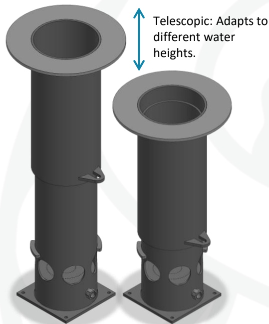
Homogenisation Air-Lifts
